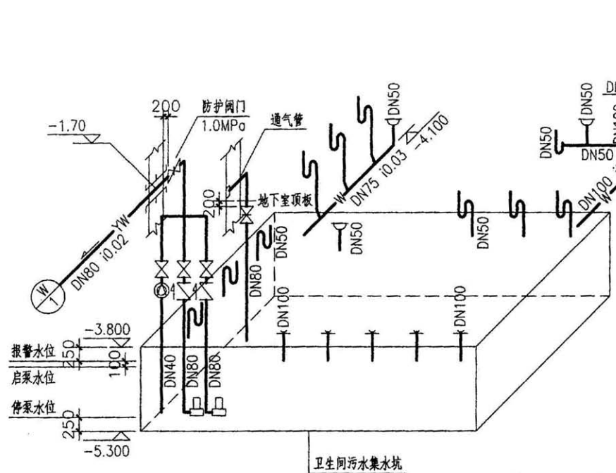
排水轴测图
