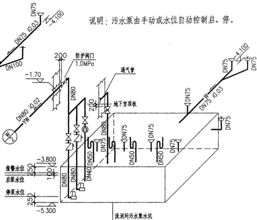
排水轴测图
