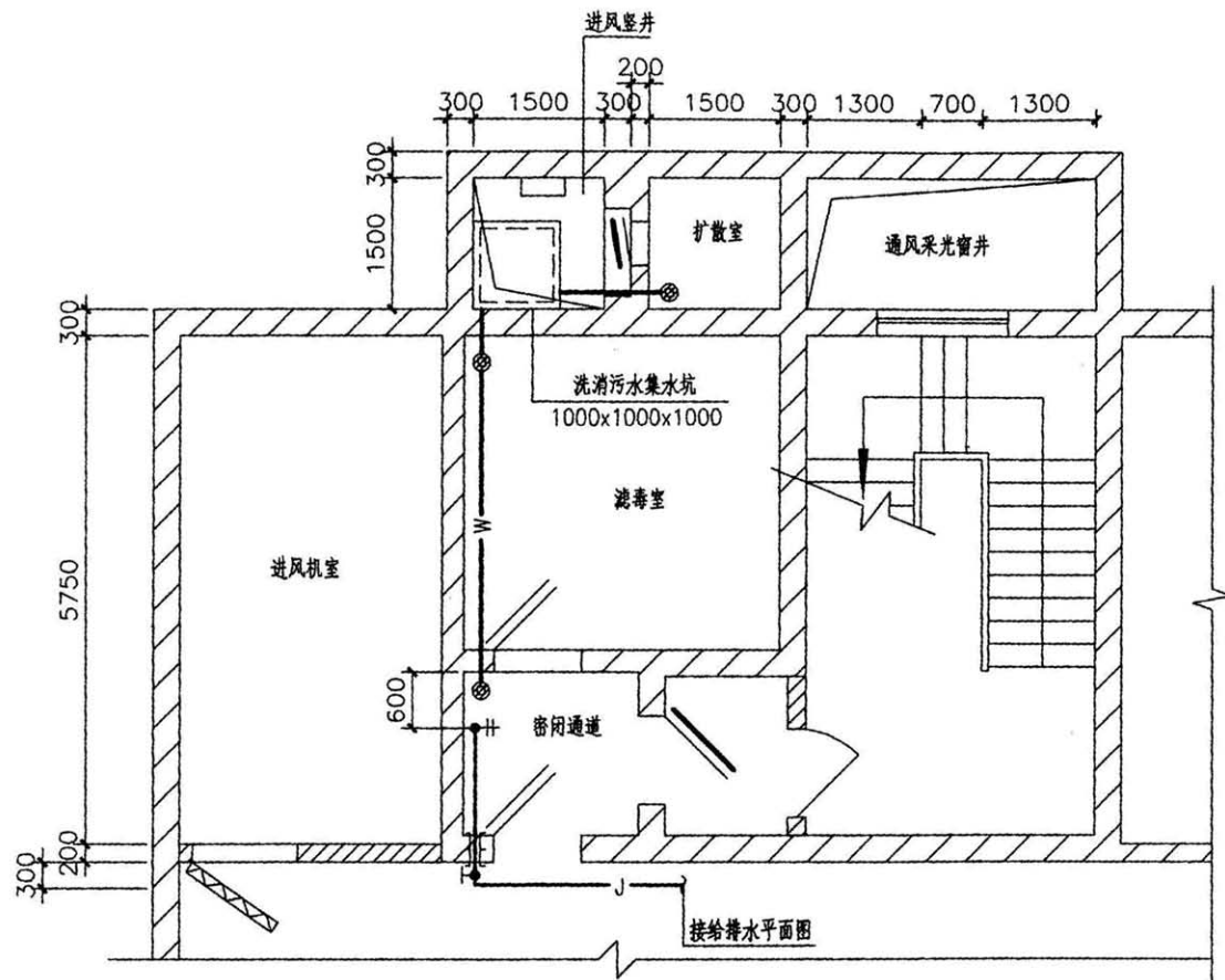
进风口部给排水放大图
